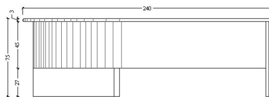
VISTA D ESC 1:25
