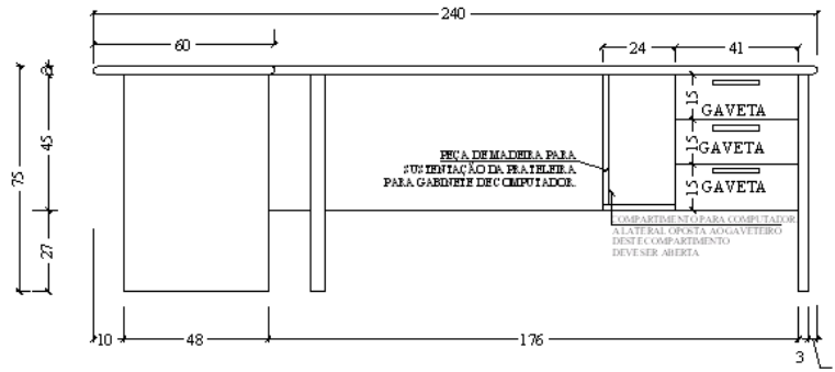
VISTA A ESC 1:25
