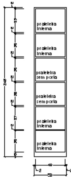
VISTA FRONTAL INTERNA ESC 1:25
