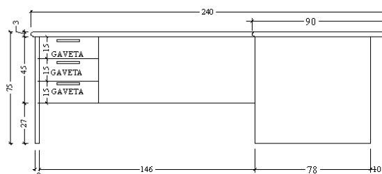
VISTA B ESC 1:25
