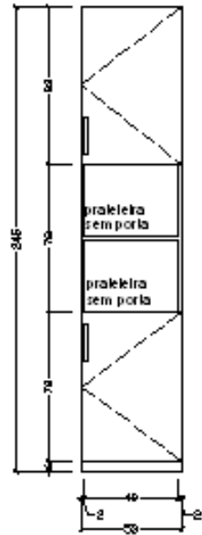
VISTA FRONTAL ESC 1:25
