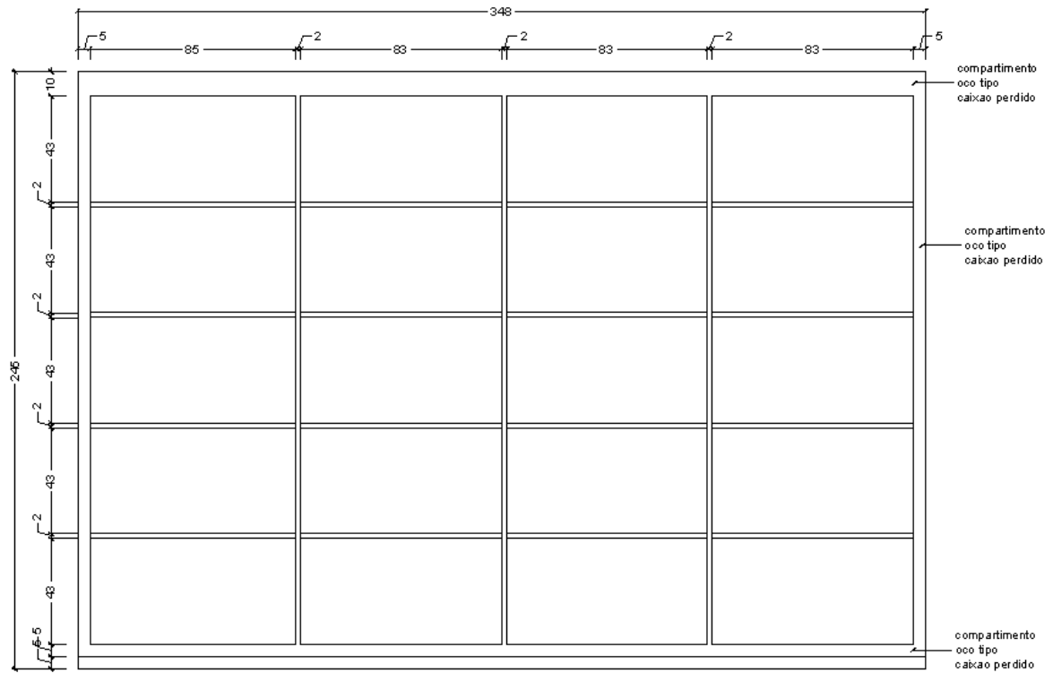
VISTA FRONTAL ESCALA: 1:25
