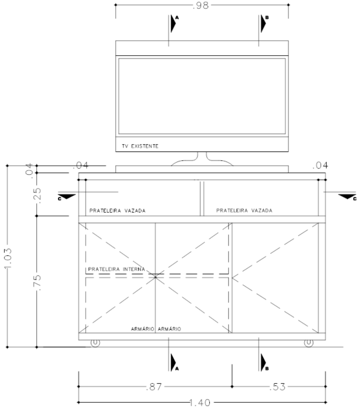
VISTA FRONTAL ESCALA 1:15
