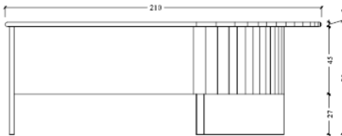
VISTA D ESC 1:25
