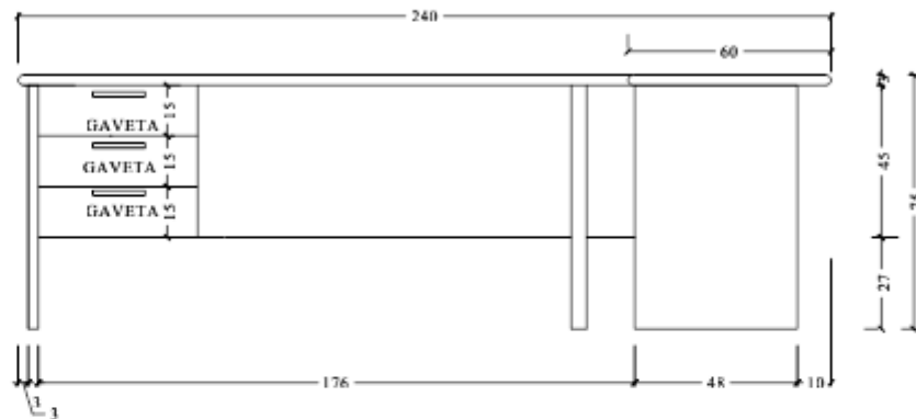
VISTA A ESC 1:25
