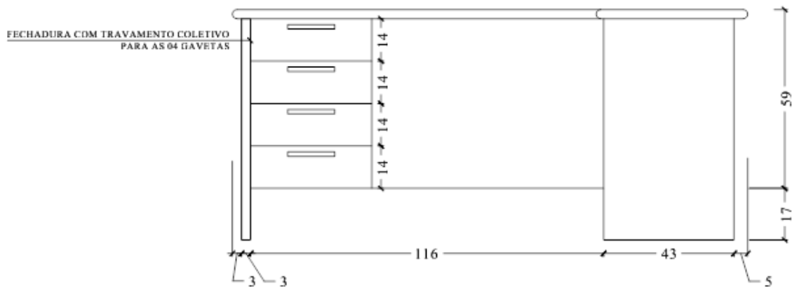
VISTA D ESC 1:20
