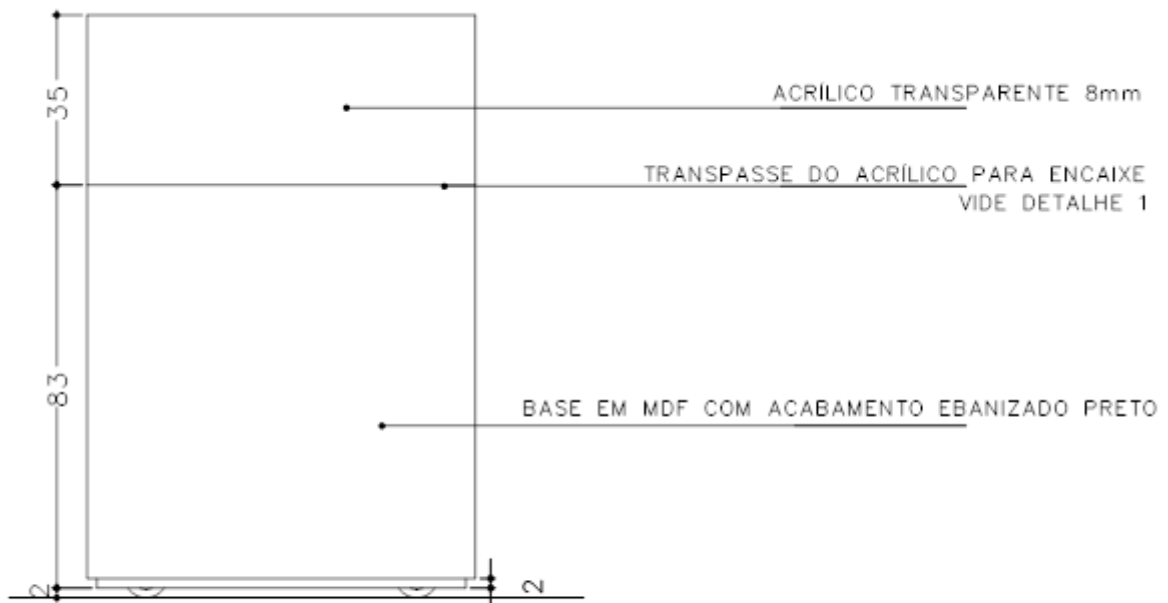
VISTA A ESCALA 1:20
