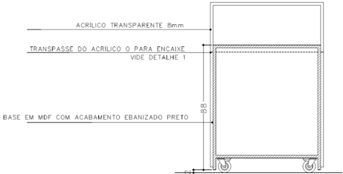
CORTA AA ESCALA 1:20
