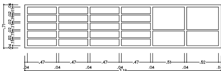
VISTA FRONTAL SEM PORTAS ESCALA: 1:20
