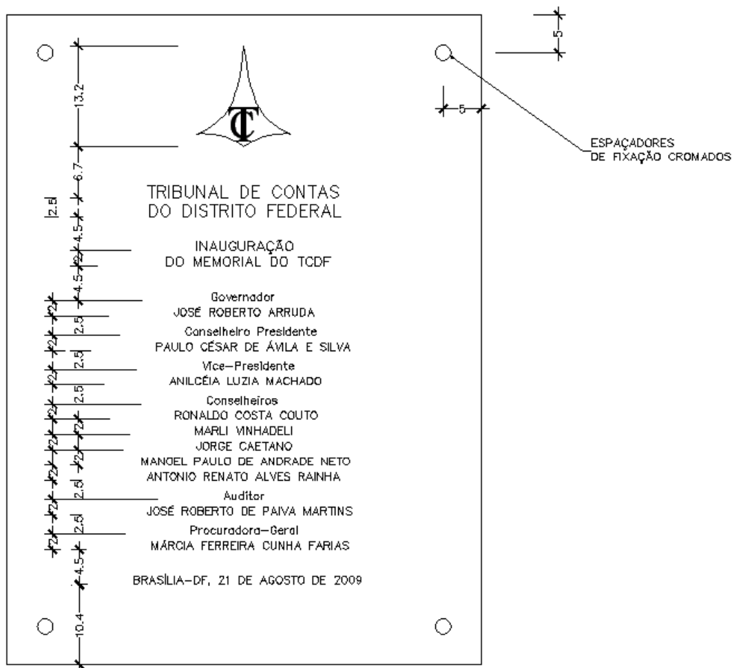
PLACA DE INAUGURAÇÃO DETALHE ESCALA 1:10
