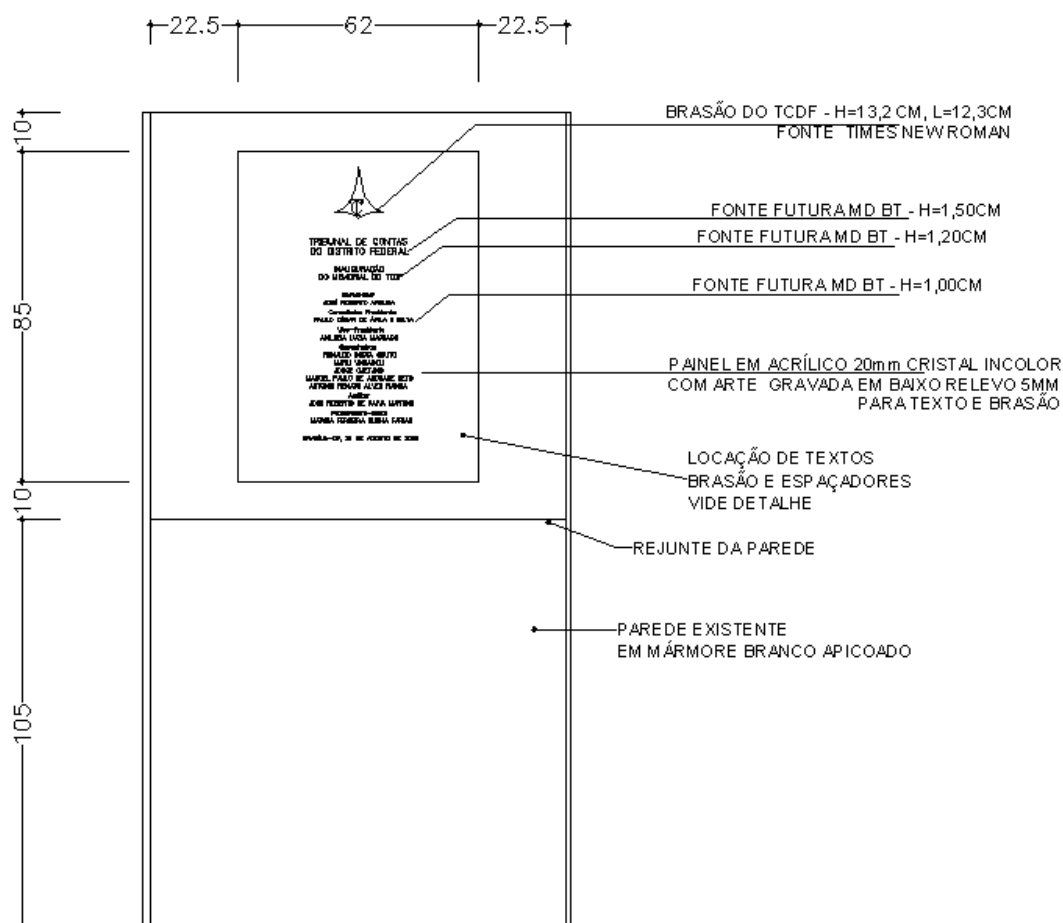
PLACA DE INAUGURAÇÃO VISTA FRONTAL ESCALA 1:20
