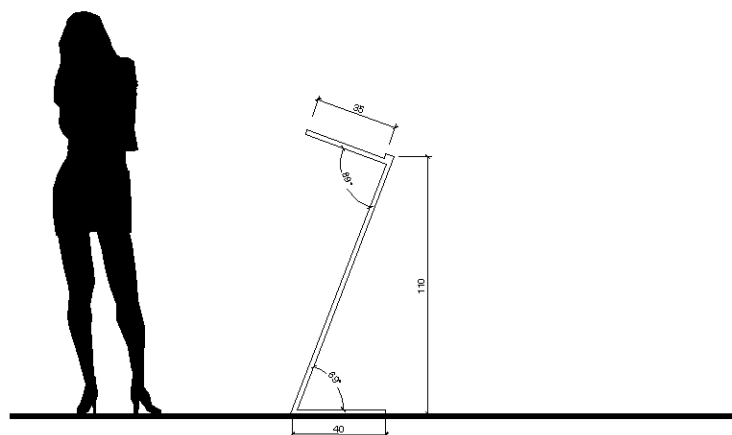
VISTA LATERAL ESC: 1/20
