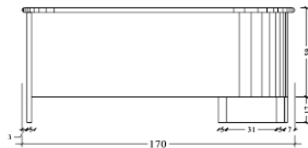
VISTA B ESC 1:20
