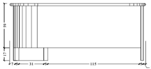
VISTA B ESC 1:20
