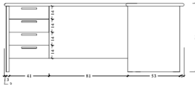
VISTA D ESC 1:20
