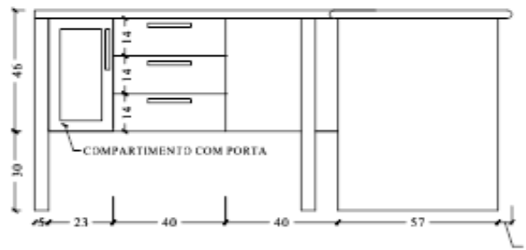
VISTA C ESC 1:20
