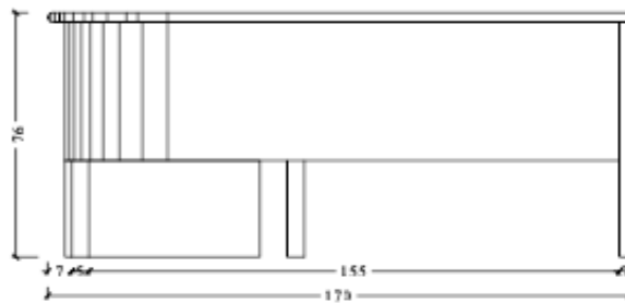
VISTA A ESC 1:20
