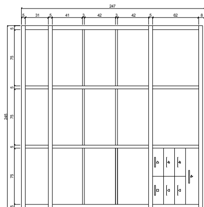
VISTA FRONTAL INTERNA ESC 1:25
