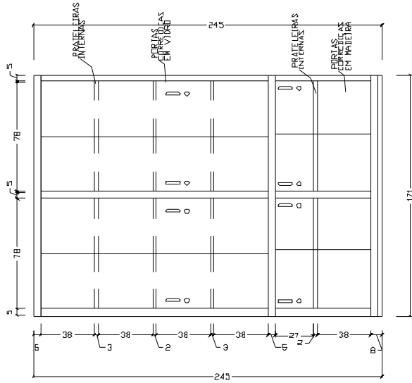
VISTA FRONTAL ESC 1:25
