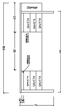
VISTA POSTERIOR ESC 1:30
