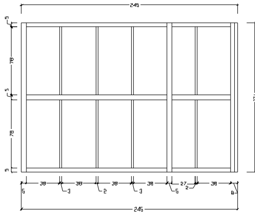
VISTA FRONTAL INTERNA ESC 1:25
