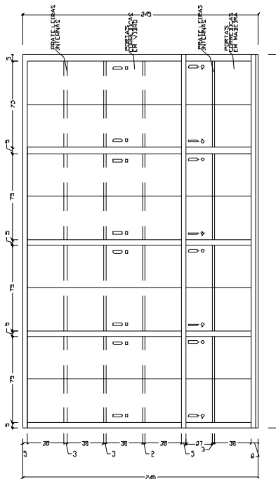
VISTA FRONTAL ESC 1:25 ESPECIFICAÇÕES
