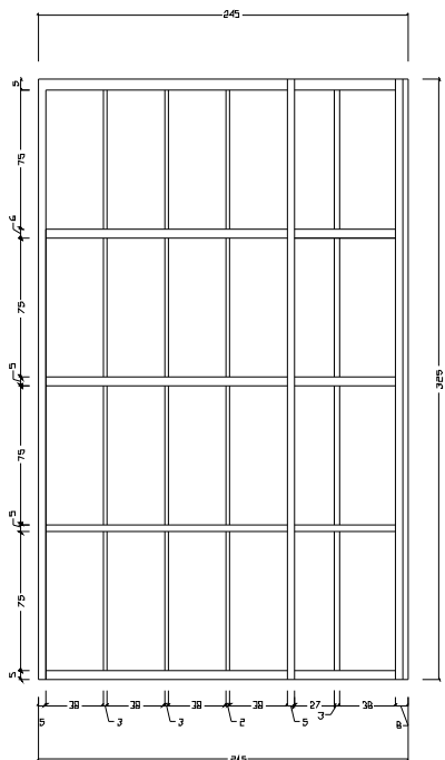
VISTA FRONTAL INTERNA ESC 1:25
